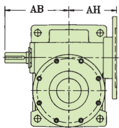
直結雙入
