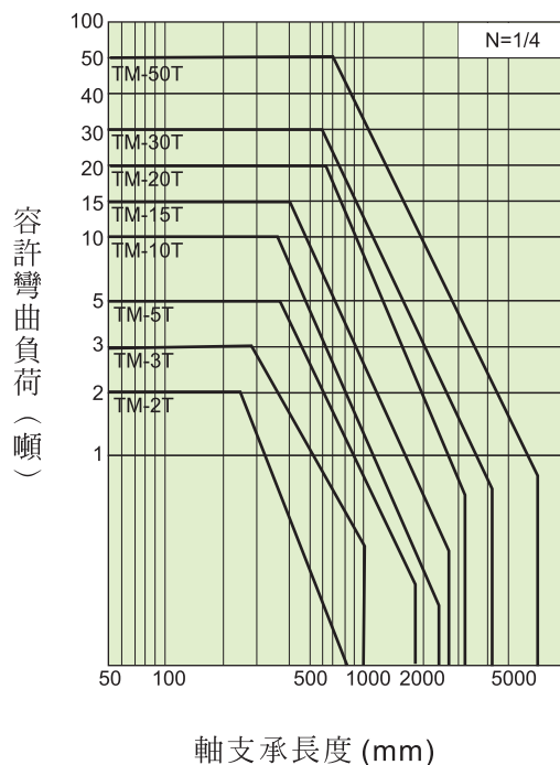
千斤頂固定一軸端游離
