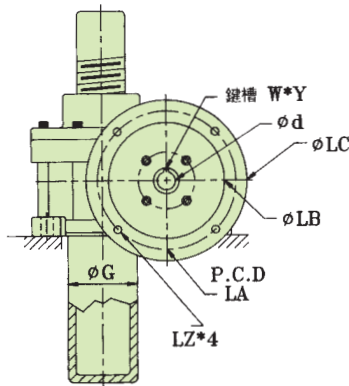
直結式
